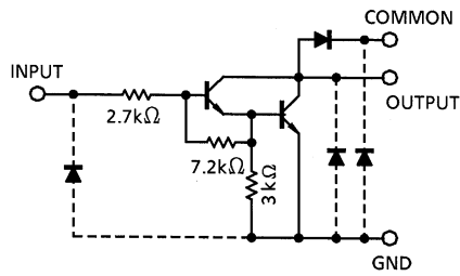
TD62003APG/AFG
