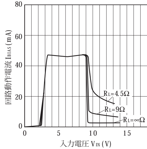
図 18 回路動作電流—入力電圧特性 (PQ09RD21)
