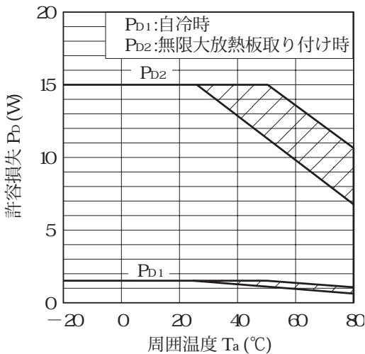
図3 許容損失低減曲線
