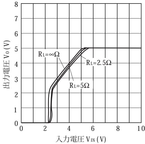
図 13 出力電圧—入力電圧特性 (PQ05RD21)
