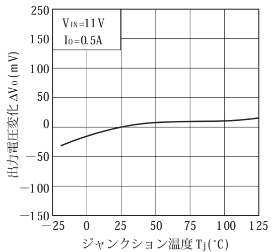
図10 出力電圧変化—ジャンクション温度特性 (PQ09RD21)
