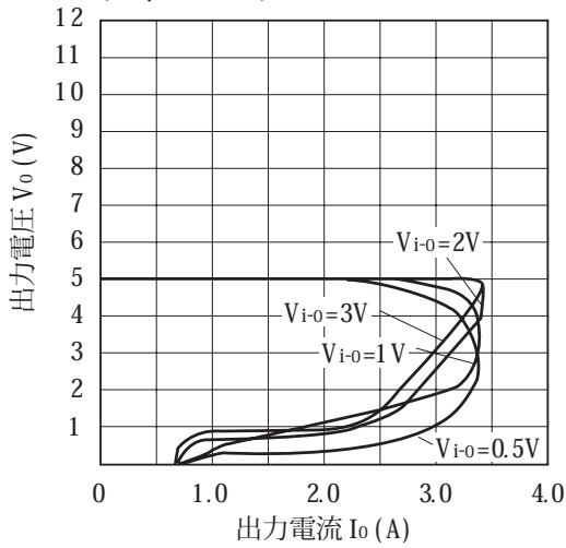
図5 過電流保護特性 (代表値) (PQ05RD21)
