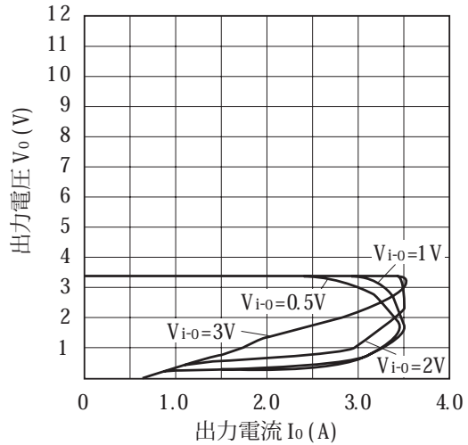
図4 過電流保護特性 (代表値) (PQ3RD23)
