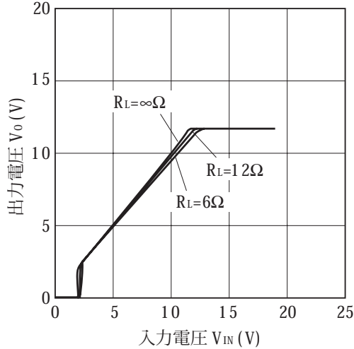
図 15 出力電圧—入力電圧特性 (PQ12RD21)
