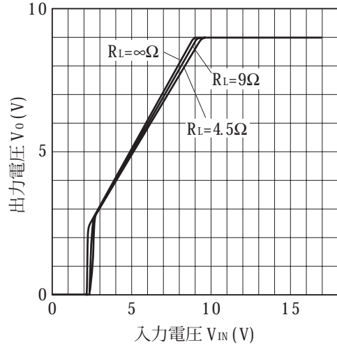
図 14 出力電圧—入力電圧特性 (PQ09RD21)
