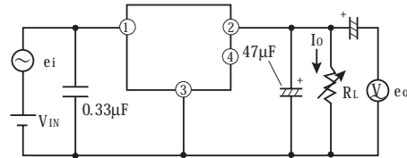
図2 リップル除去率測定回路
