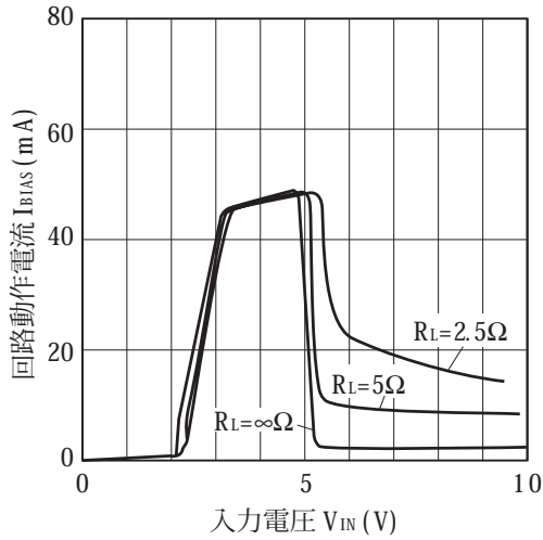
図 17 回路動作電流—入力電圧特性 (PQ05RD21)
