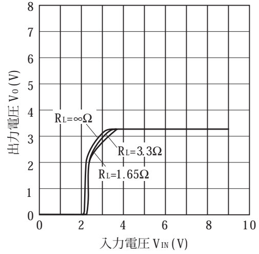
図 12 出力電圧—入力電圧特性 (PQ3RD23)
