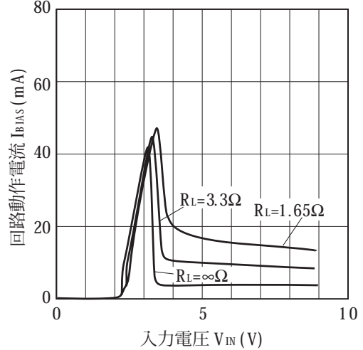
図 16 回路動作電流—入力電圧特性 (PQ3RD23)
