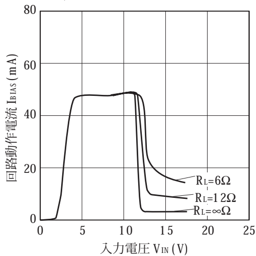
図 19 回路動作電流—入力電圧特性 (PQ12RD21)
