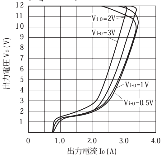
図7 過電流保護特性 (代表値) (PQ12RD21)
