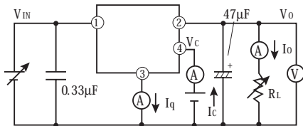
図1 レギュレータ標準測定回路
