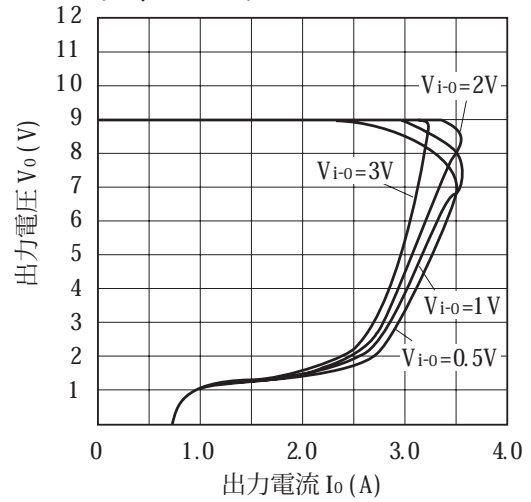
図6 過電流保護特性 (代表値) (PQ09RD21)
